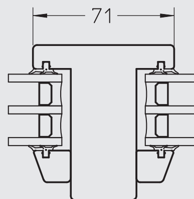
HORISONTALSNITT
