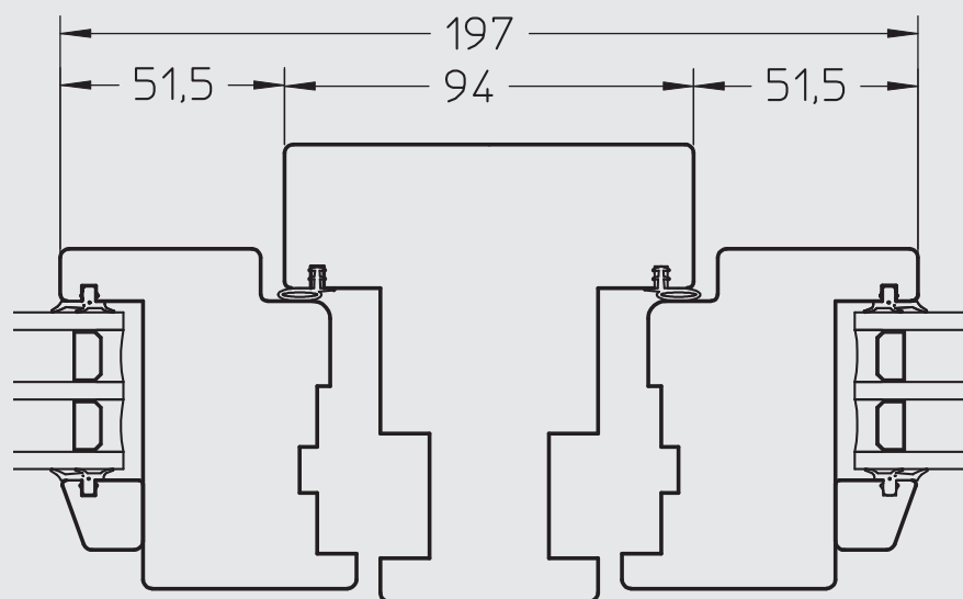
HORISONTALSNITT
